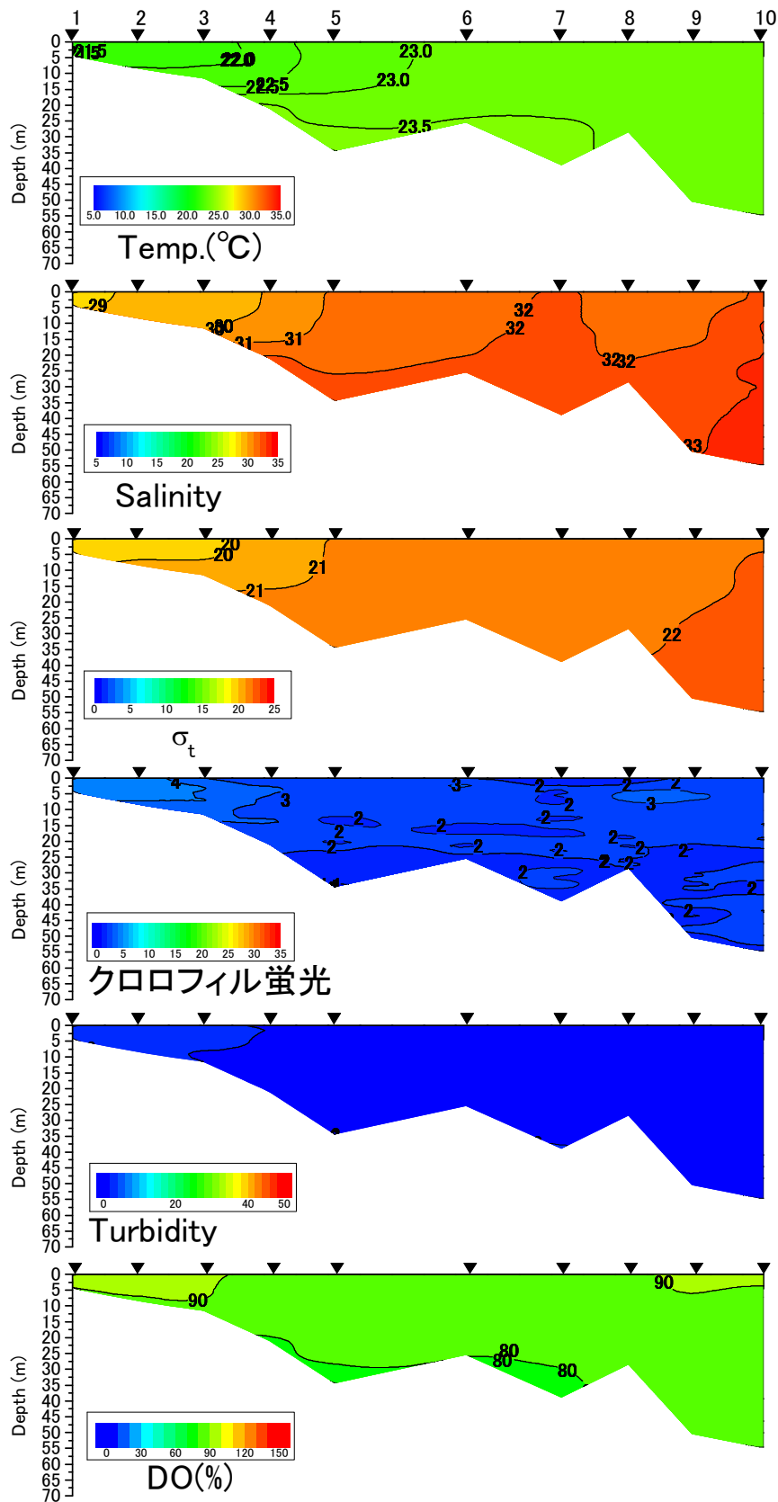
有明海中央ラインの水温(°C)、塩分、密度( \sigma_t )、クロロフィル蛍光強度、濁度、溶存酸素飽和度(DO%)の鉛直面図(国土交通省の調査による) (2016年10月24日)
